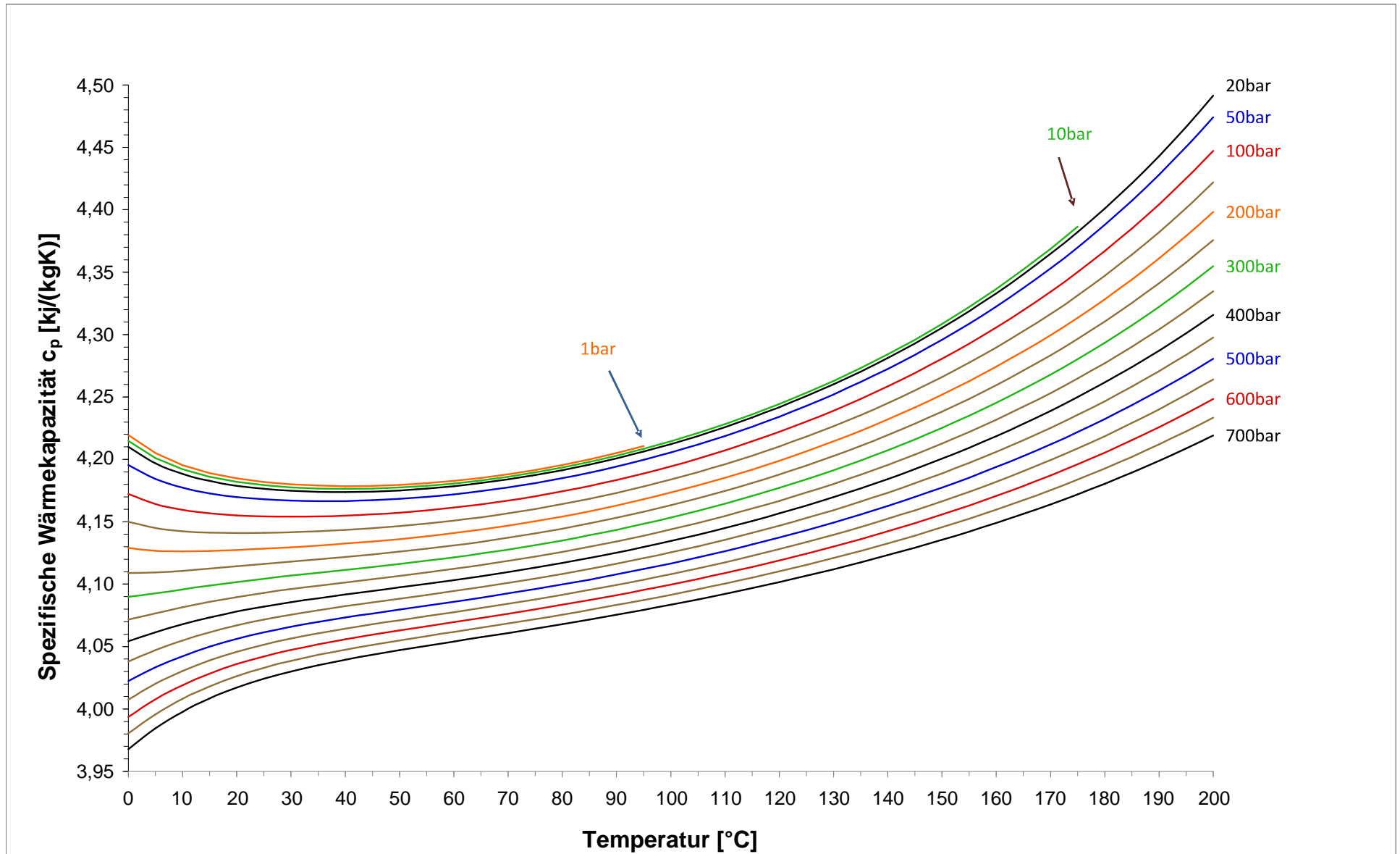
Abhängigkeit der spezifischen Wärmekapazität reinen Wassers von Druck und Temperatur, nach Wagner & Kretschmar (2008)
